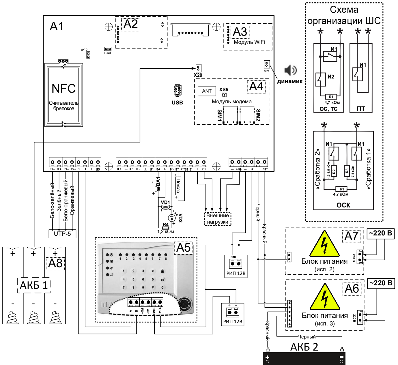
Рисунок 6 – Схема подключения
