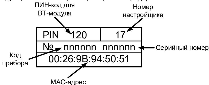
Рисунок 34 – Шильдик на плате КОП-02.6, -04, -05
