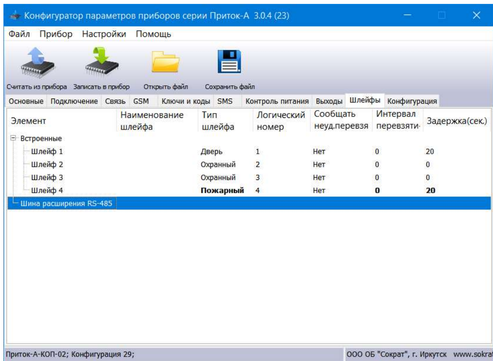
Рисунок 18 – Вкладка «Шлейфы»
