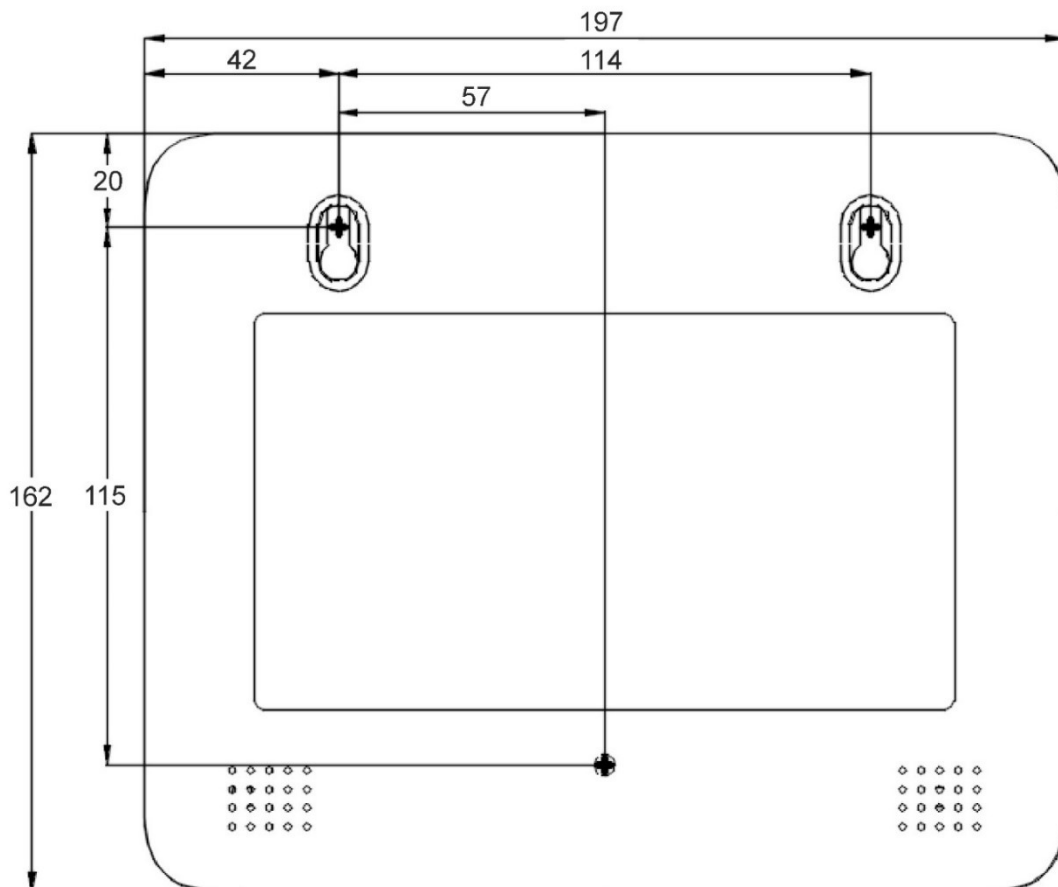
Рисунок 56 – Разметка отверстий для крепления прибора КОП-02.6, КОП-01 исп.1 и КОП-04 (вид со стороны передней панели)
