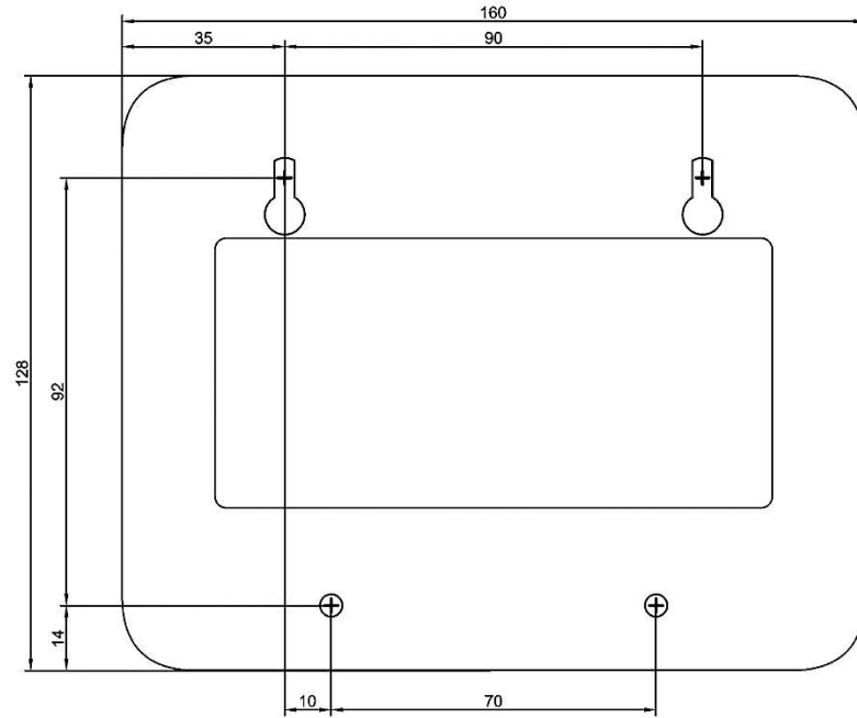
Рисунок 58 – Разметка отверстий для крепления прибора КОП-02.4 (вид со стороны передней панели)
